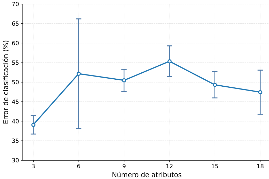
Figura 5: Error de clasificación de la tubería suplementaria de regresión logística con SMOTE en función del número de atributos seleccionados por ganancia de información dentro de Training . Las barras de error representan la variabilidad reportada para cada validación cruzada estratificada de 10 particiones.
